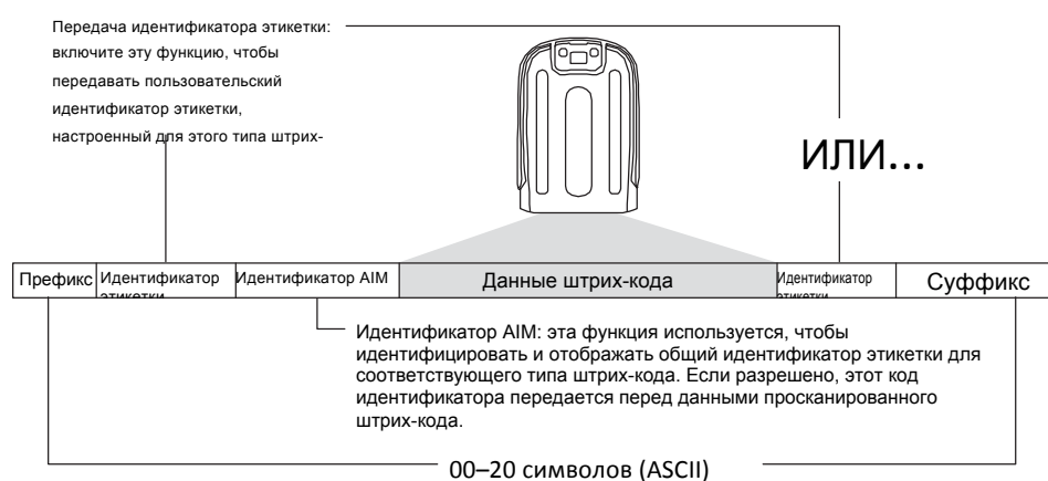
Рис. 7. Структура строки сообщения
