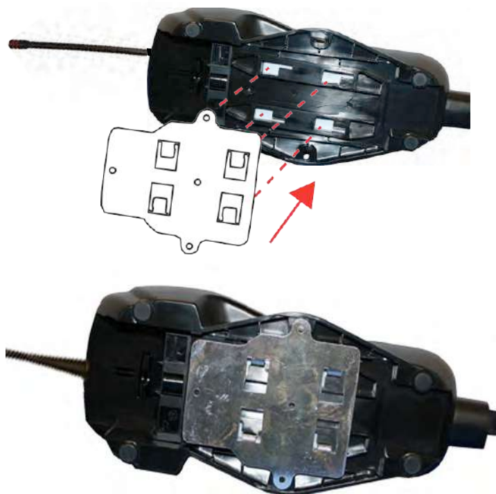
Базовая станция с прикрепленной монтажной пластиной
