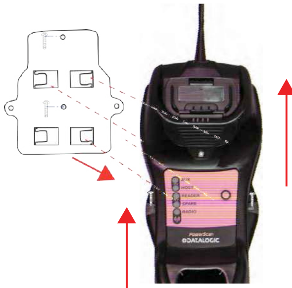
Рис. 4. Монтаж пластины на стене
